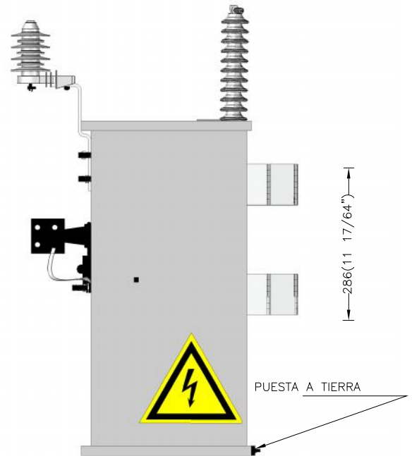
VISTA LATERAL DERECHA ESC. SIN
