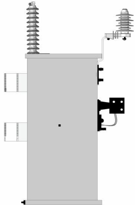
VISTA LATERAL IZQUIERDA ESC. SIN
