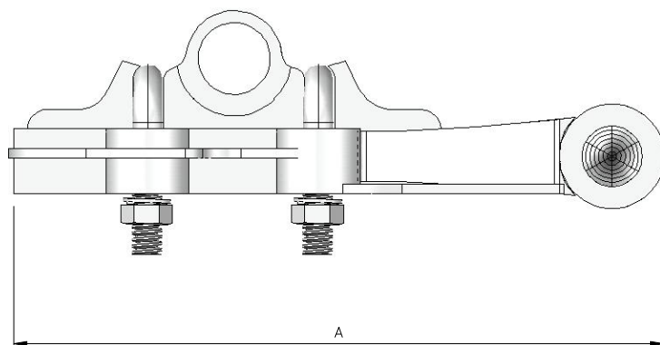
VISTA LATERAL escala 1:2
