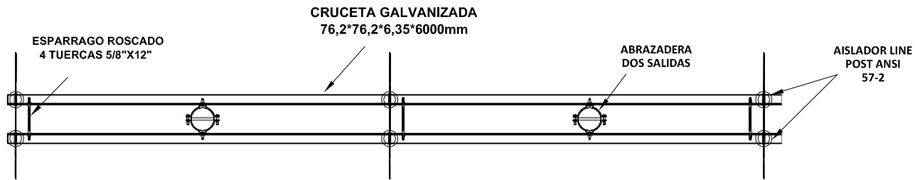
VISTA PLANTA
