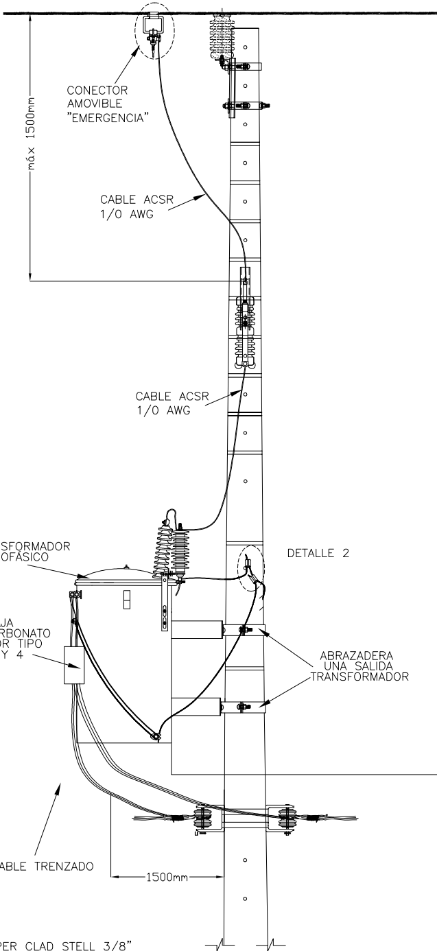
DETALLE 1
