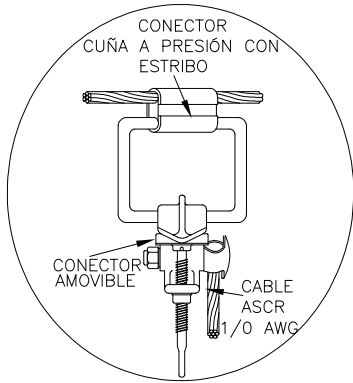
DETALLE 1 CONEXION A RED MT
