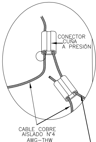
DETALLE 2 CONEXION TIERRA COOPER CLAD
