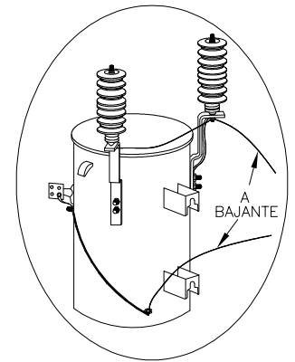
VISTA ISOMETRICA CONEXION TIERRA DPS
